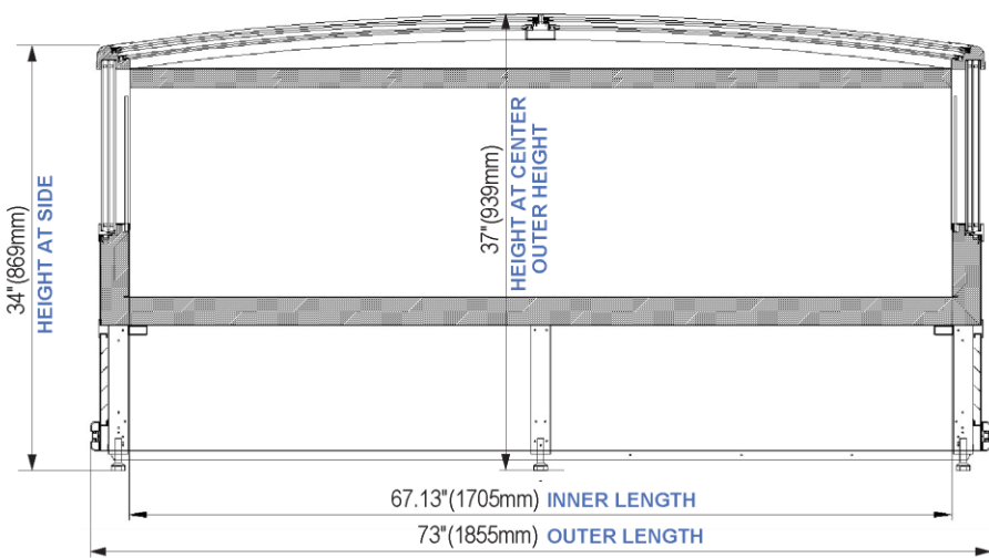
Longitudinal Section:
