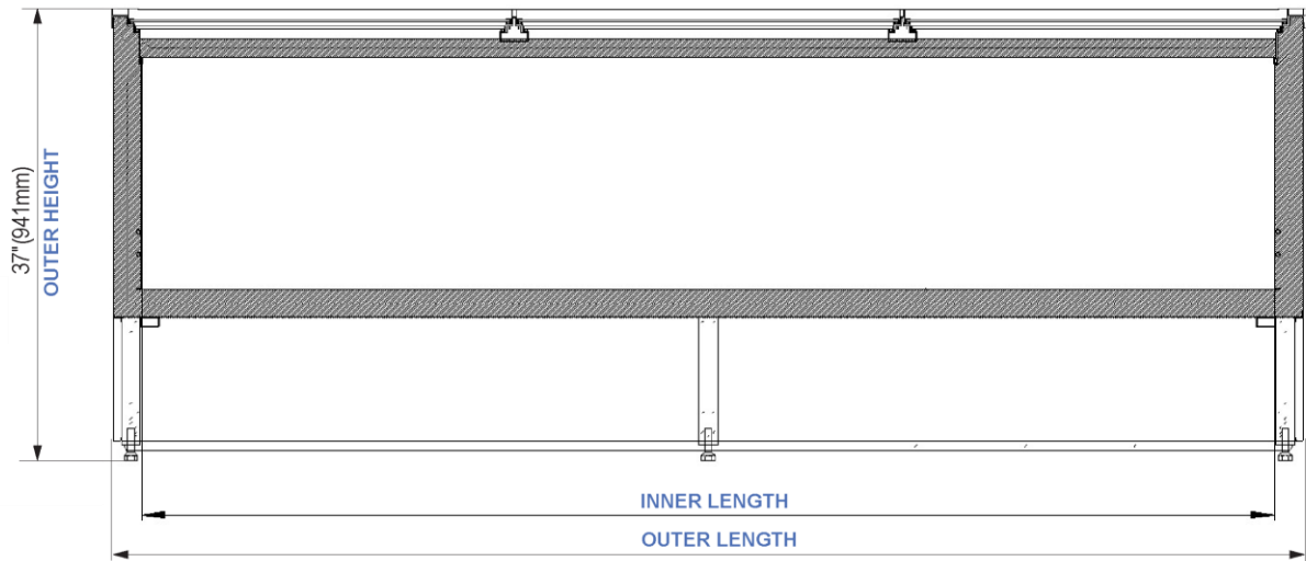
Longitudinal Section:
